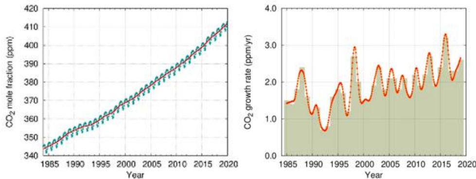
Abb. 2: Globaler durchschnittlicher CO 2 -Gehalt in der Atmosphäre (links) und die Wachstumsrate (rechts) von 1984 bis 2019 9
